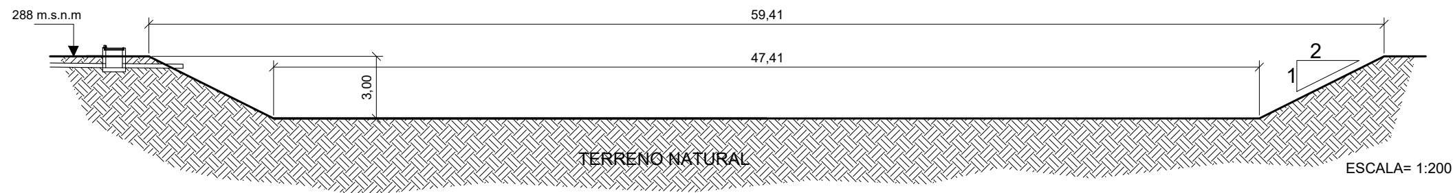
CORTE ESCALA= 1:200
